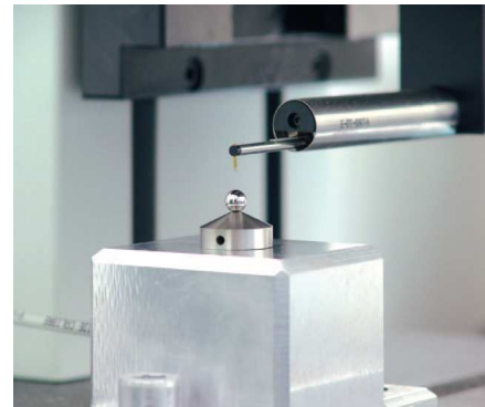
Mesure de la rugosité Marque : Surfcom 1500
